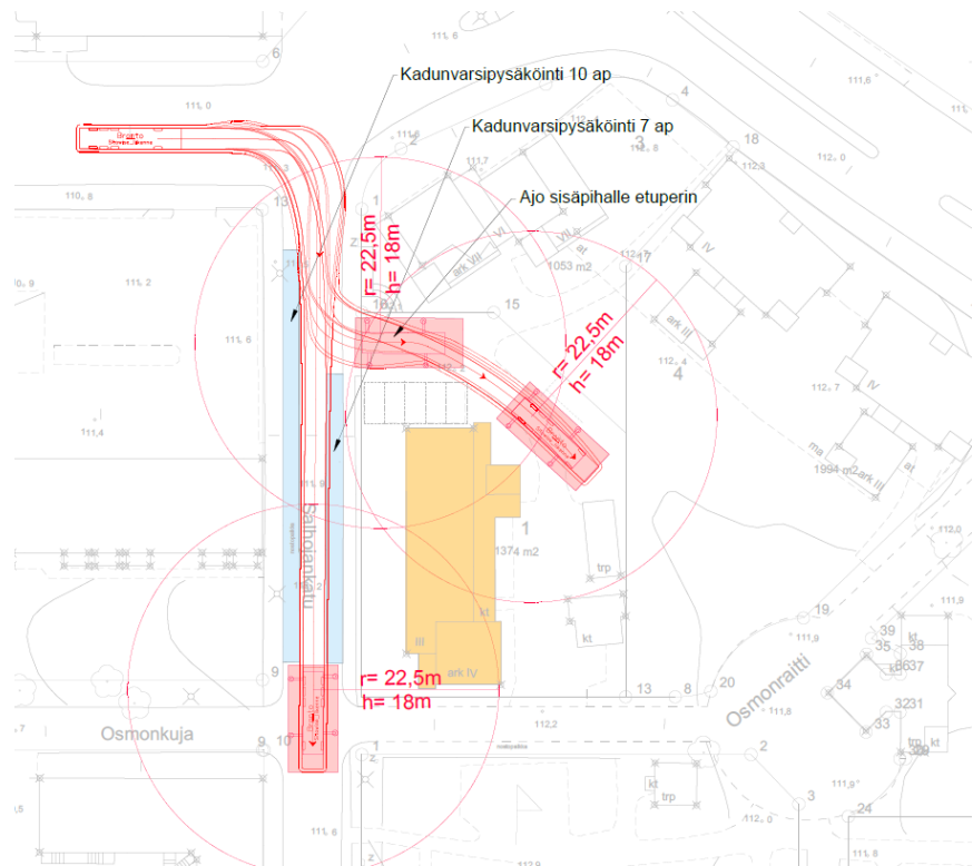
Pelastusajoneuvon ajouratarkastelu nykytilanteessa, WSP 2022
