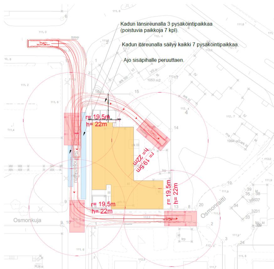
Pelastusajoneuvon ajouratarkastelu kaavan suunnitteluratkaisussa, WSP 2022
