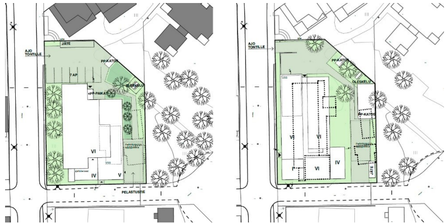
Vasemmallalla on asemapiirros säilyttävästä vaihtoehdosta, oikealla asemapiirros uudistavasta vaihtoehdosta.
